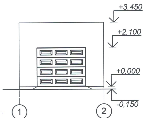
Фасад 1-2
