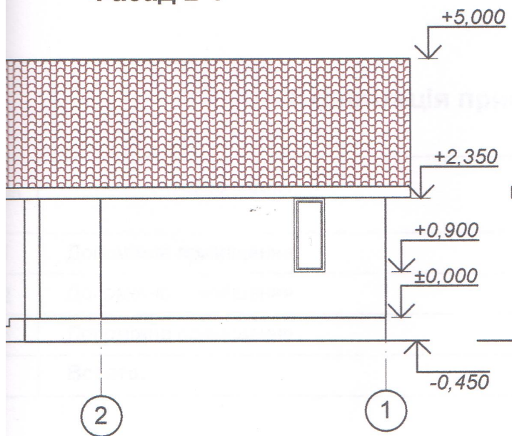
Фасад 2-1
