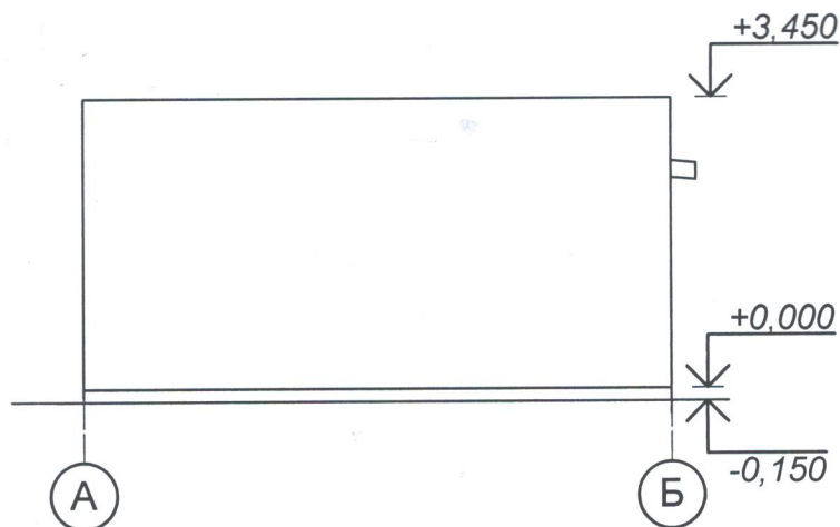
Фасад А-Б
