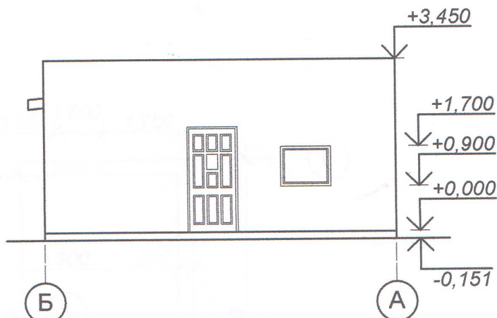
Фасад Б-А
