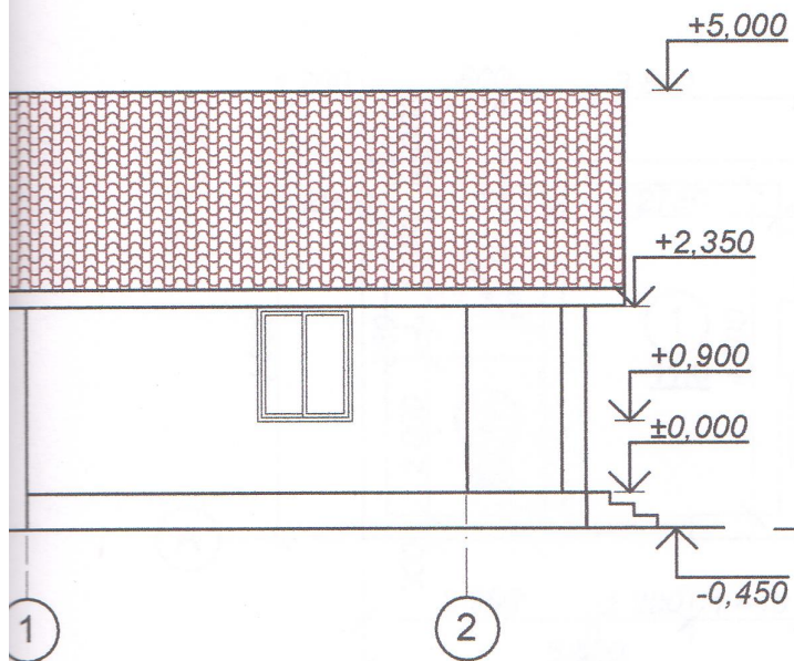
Фасад 1-2
