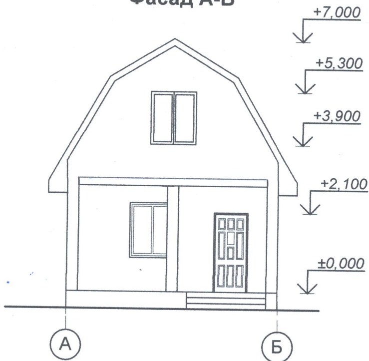
Фасад А-Б
