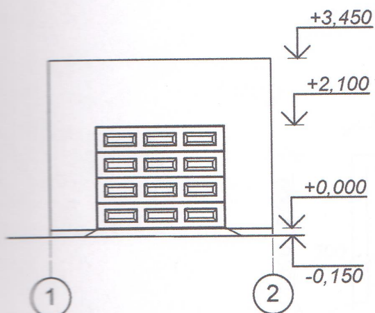
Фасад 1-2
