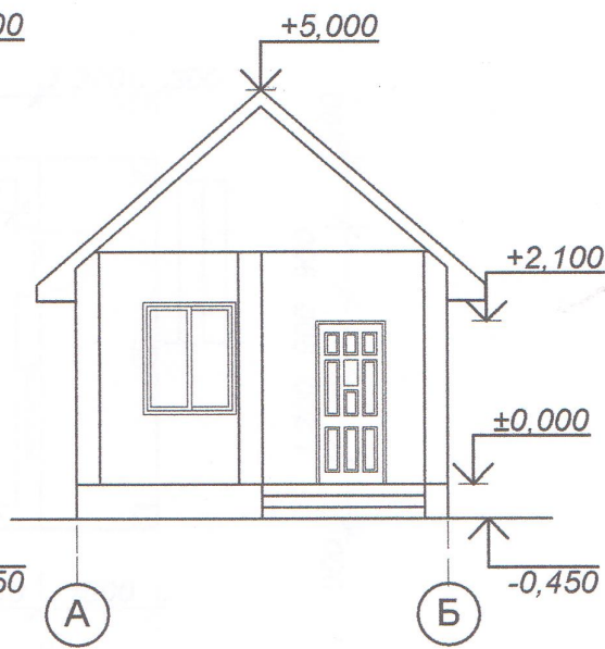
Фасад А-Б
