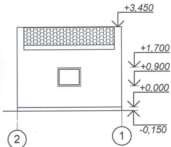
Фасад 2-1
