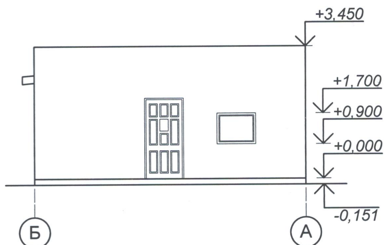
Фасад Б-А
