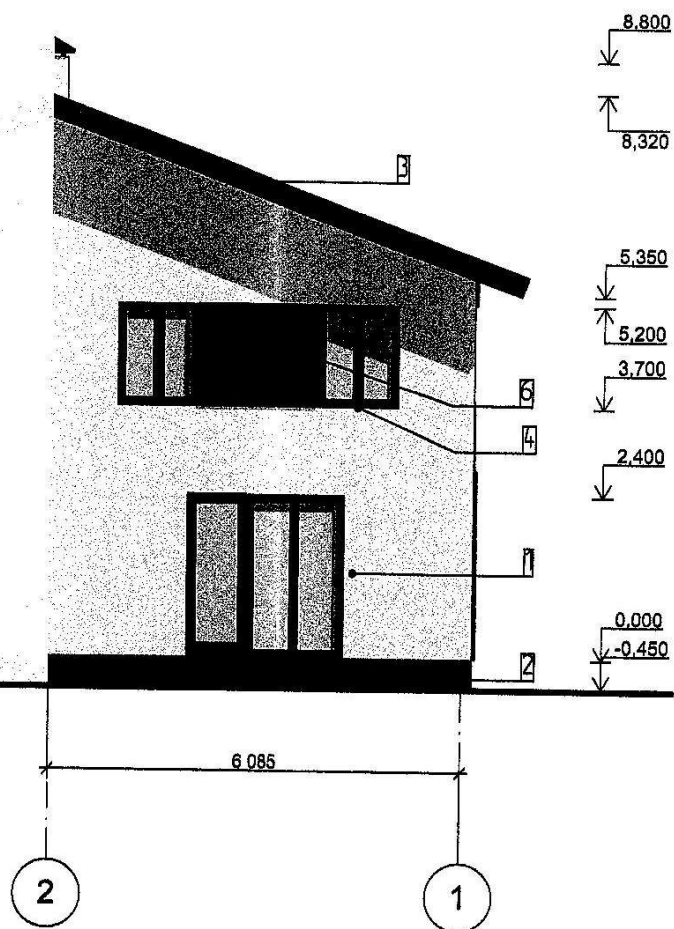
Фасад 2-1 М 1:100
