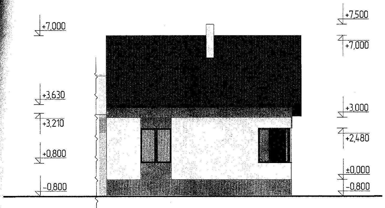
Фасад Б-А
