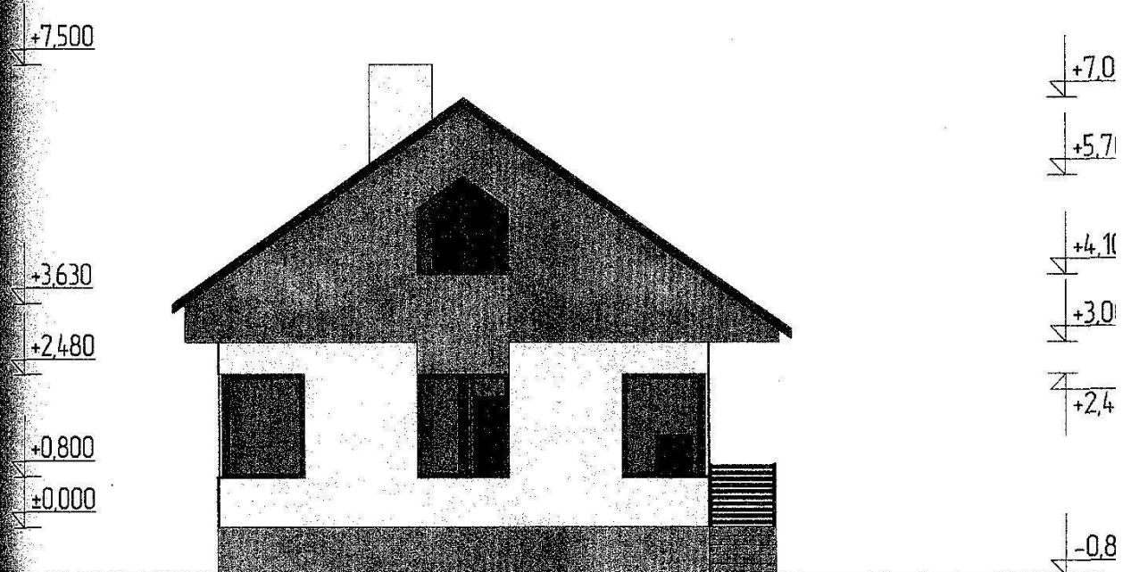
Фасад 1-2
