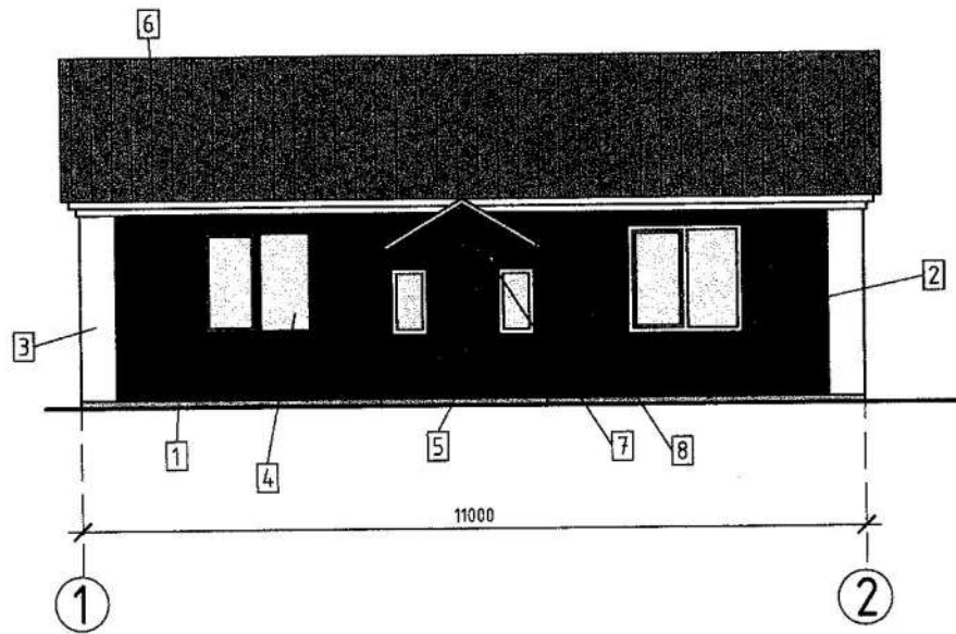
Фасад Б-А
