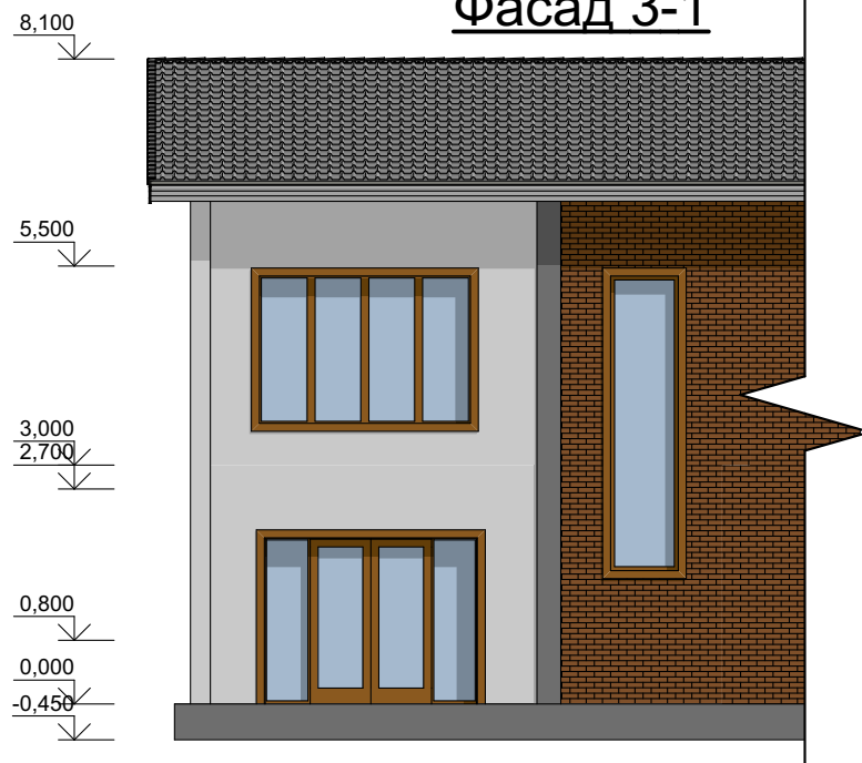
Фасад 3-1
