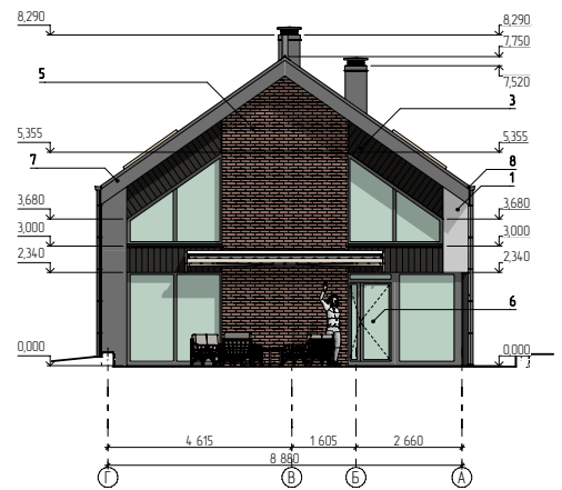
Фасад Г-А М1:100
