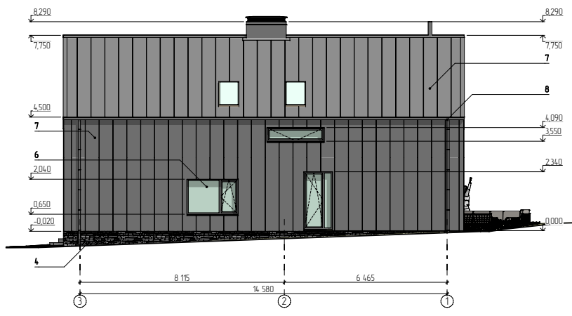
Фасад 3-1 М1:100
