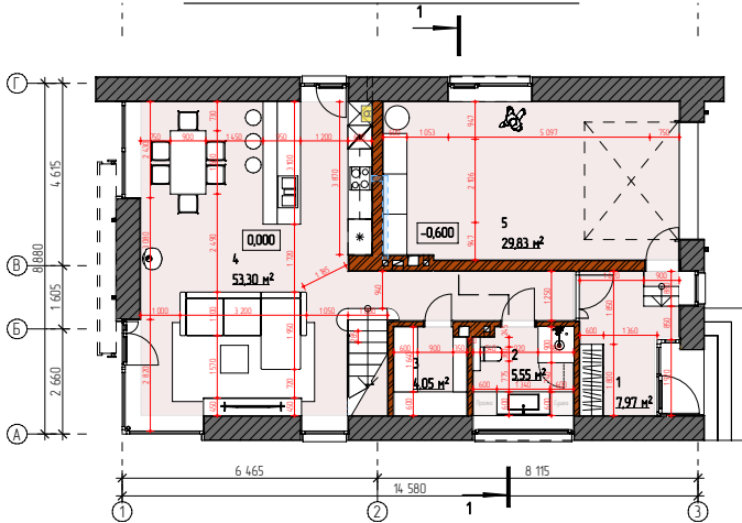
План 1-го пов. М1:100
