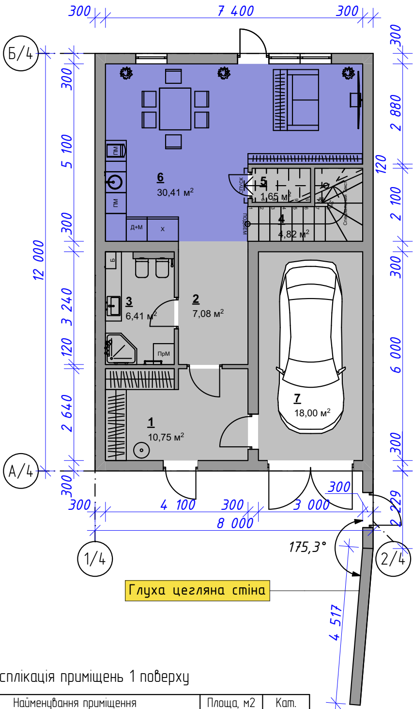
План 1 поверху , М1:100
