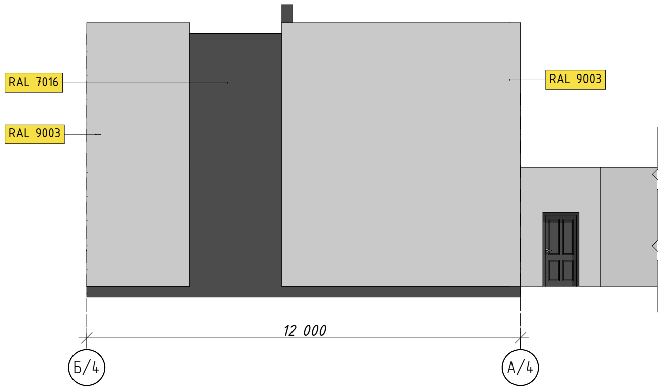
Фасад Б/4-А/4, М1:100
