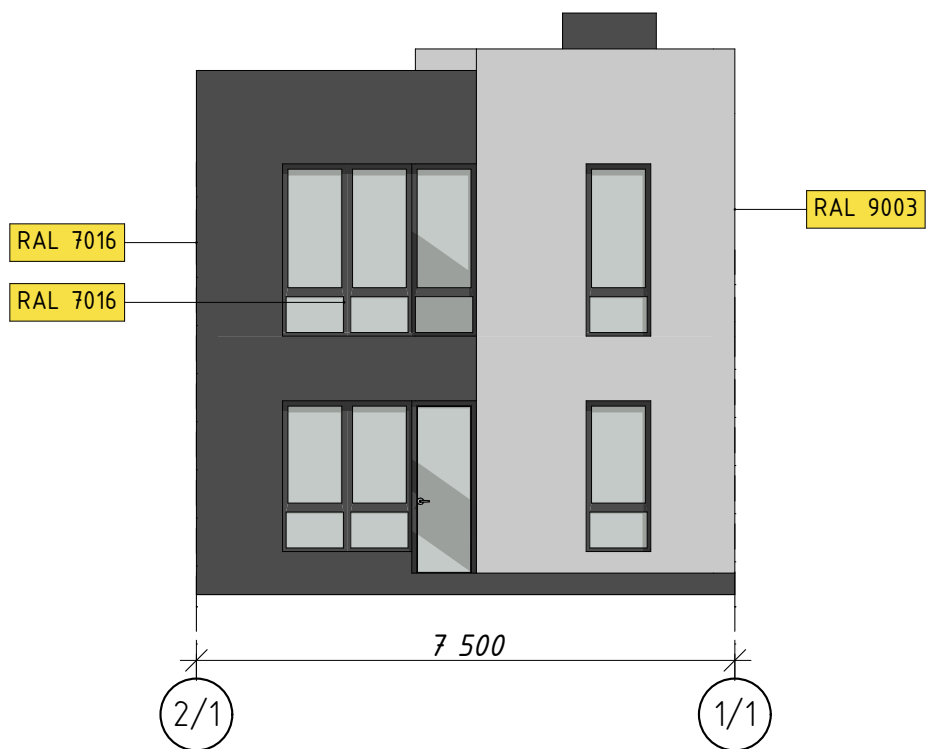
Фасад 2/1-1/1, М1:100
