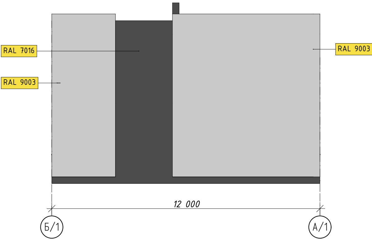
Фасад Б/1-А/1, М1:100
