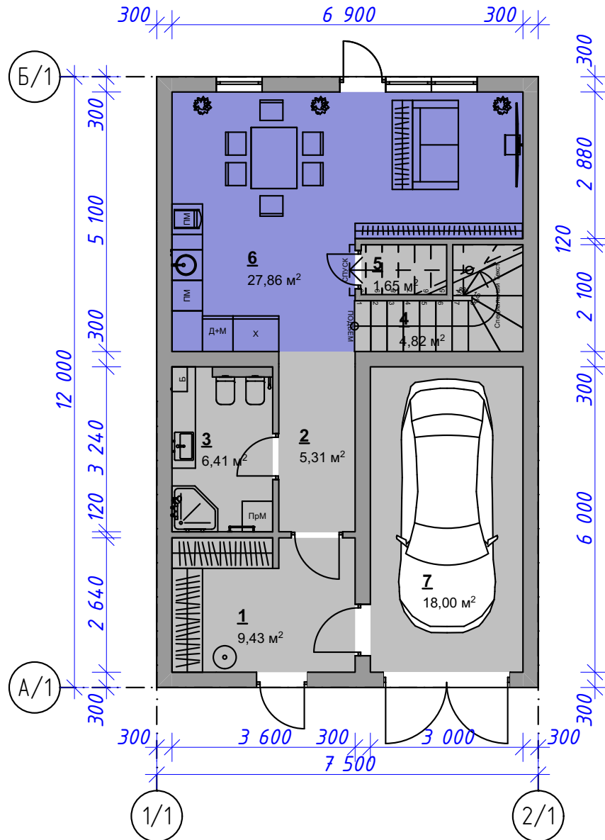
Експлікація приміщень 1 поверху
